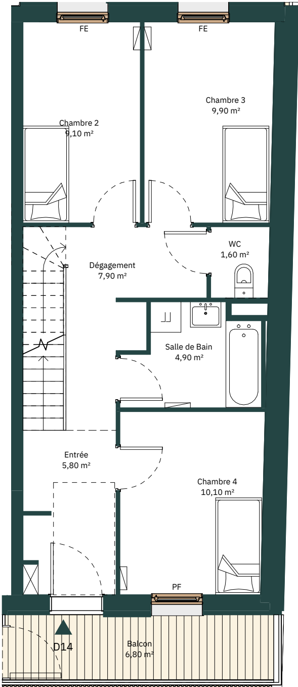
Niveau 0 - 2e étage
