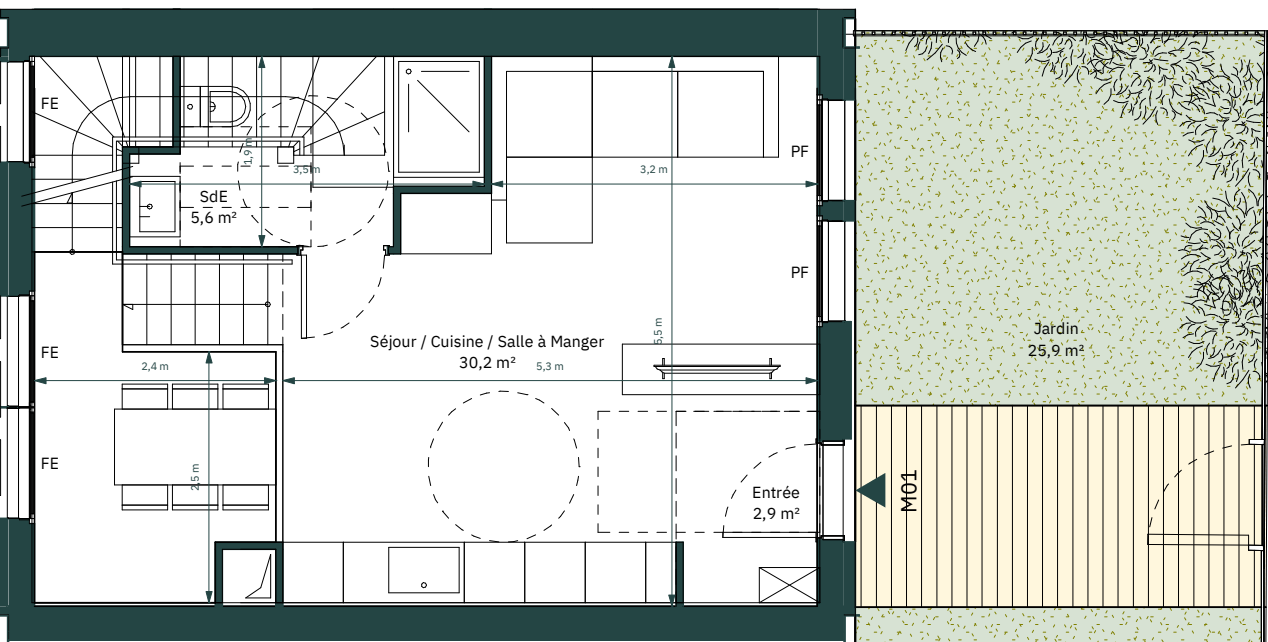
Niveau 0 - RDC
